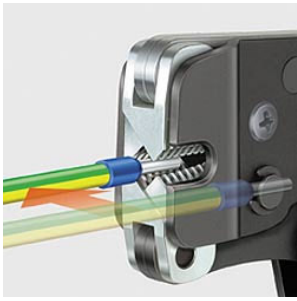
97 53 08: Indføring af kabeltyller parallelt fra siden op til 2,5 mm 2 f.eks. ved trange pladsforhold
