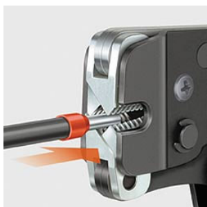
Kabeltyllerne føres forfra ind i f.eks. styreskabe
