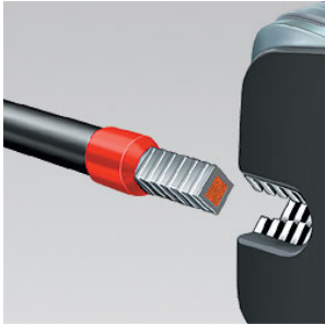
Firkant-crimping for optimale kontaktflader
